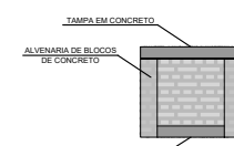
DETALHE DA CAIXA DE DRENAGEM ESC.: 1/10 (EM cm)
