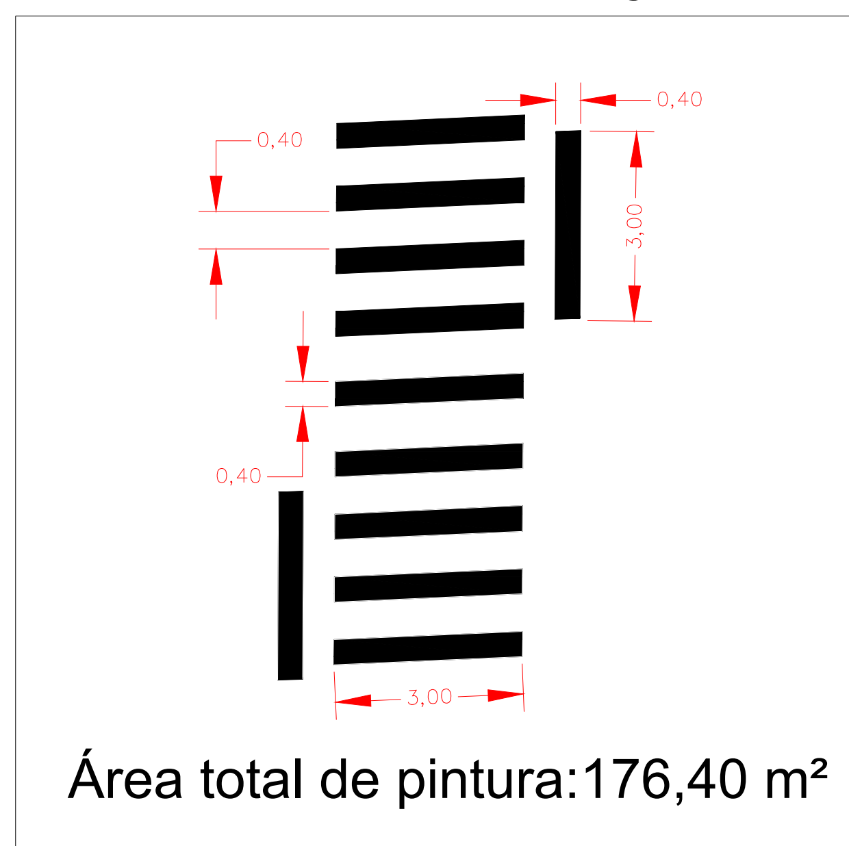
Detalhe Faixa de Segurança
